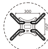
VESA 300x200
