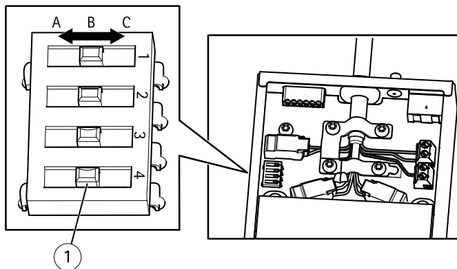
1 DIP-Schalter (4x)
