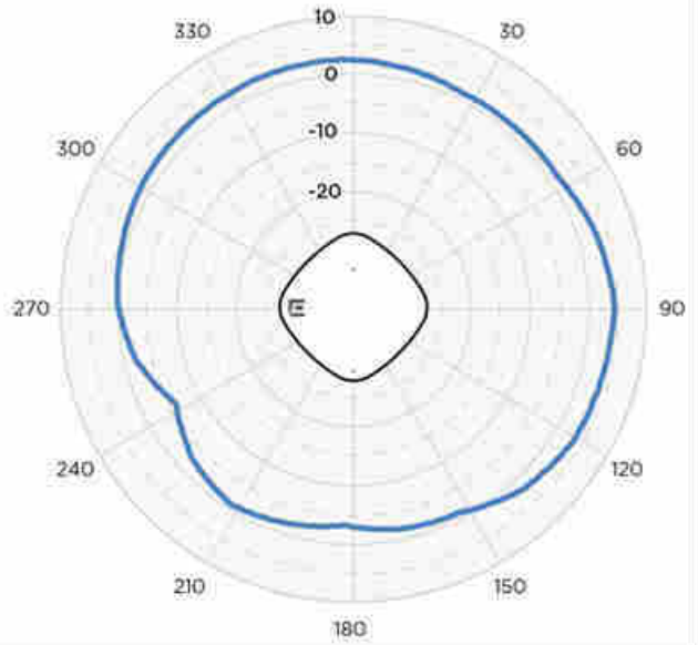
BLE Azimuth
