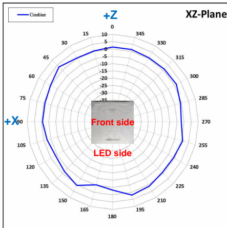
5 GHz Antenna
