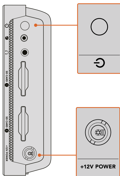
外部電源を+12V電源入力に接続。 電源ボタンを押すと、電源がオンになります。
