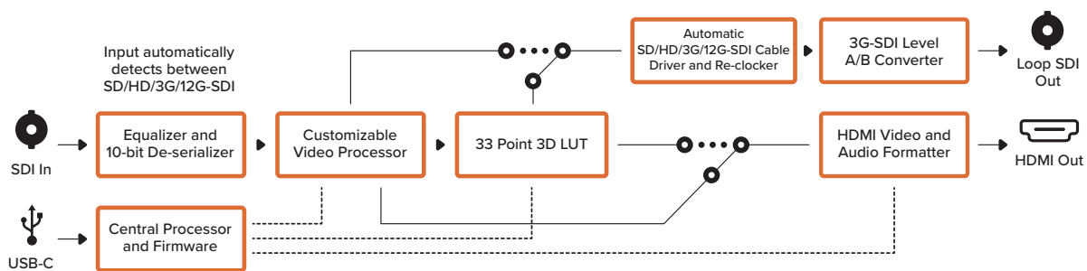
Схема соединений Micro Converter SDI to HDMI 12G
