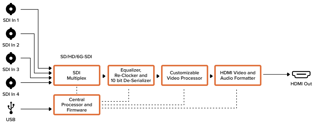
Mini Converter Quad SDI to HDMI 4K原理图
