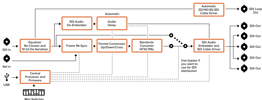
Mini Converter UpDownCross原理图
